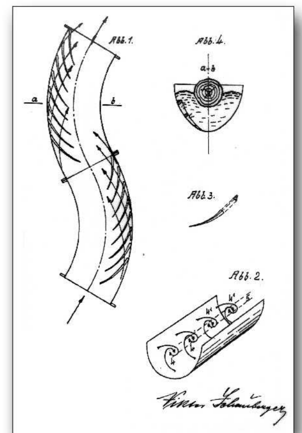
Zeichnung eines künstlichen Gerinnes
